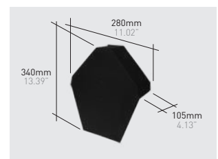
Q147*K | End cap 45° klinker
