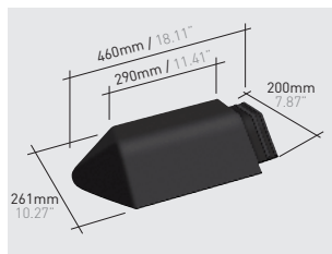
Q109*K | Atica 120° hip / end ridge klinker
