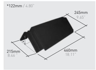
Q145*K | Ridge 45° klinker
